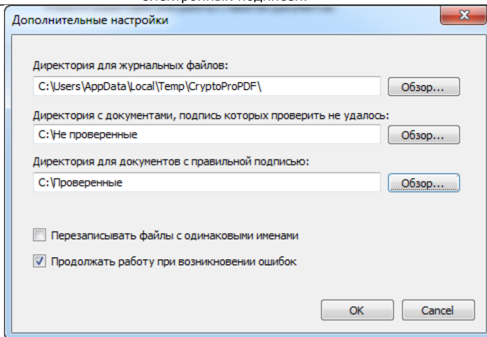
Рисунок 15. Дополнительные настройки
