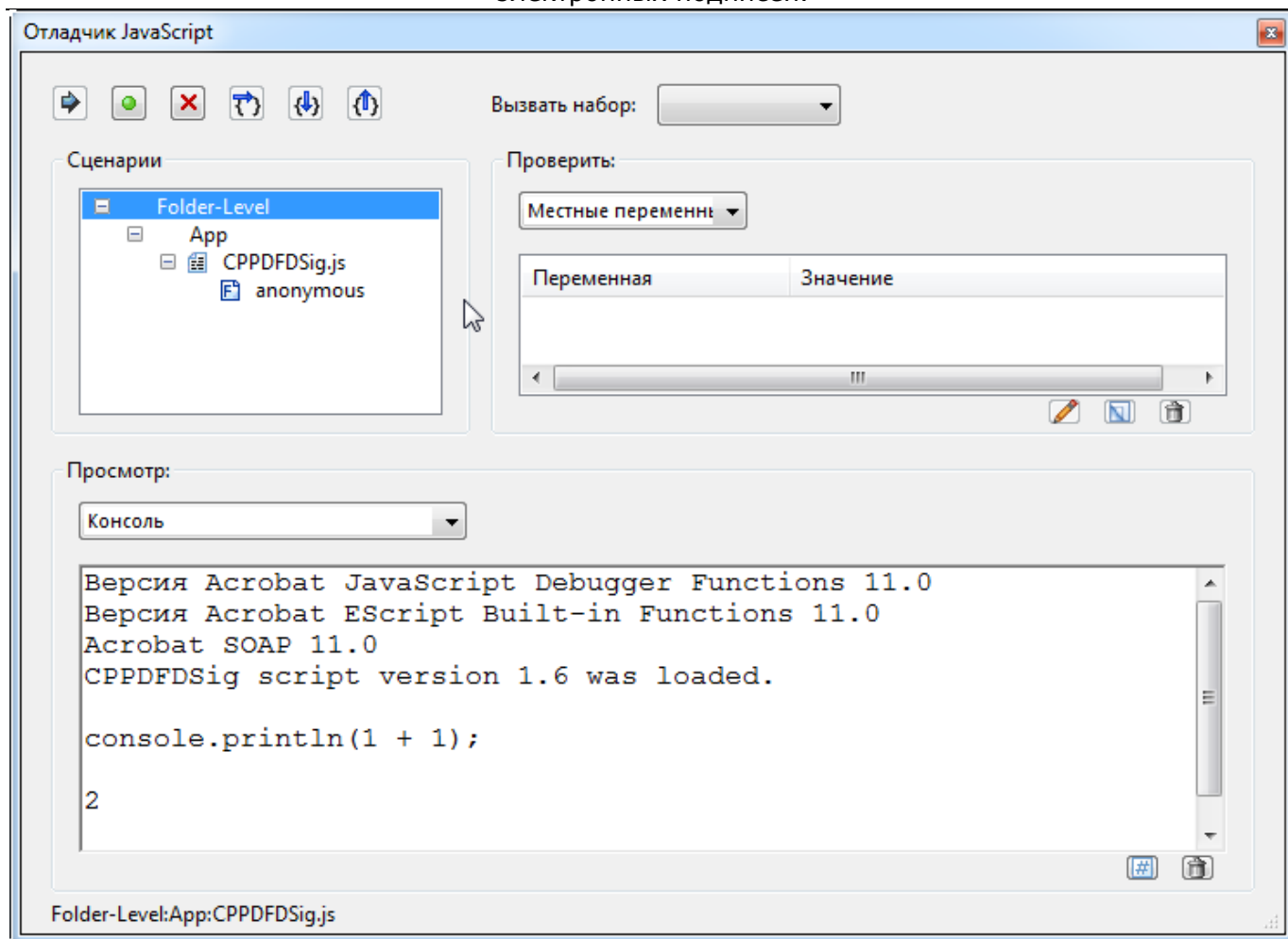
Рисунок 21. Отладчик JavaScript
