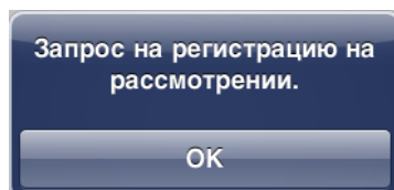
Рис. 27. Статус запроса
